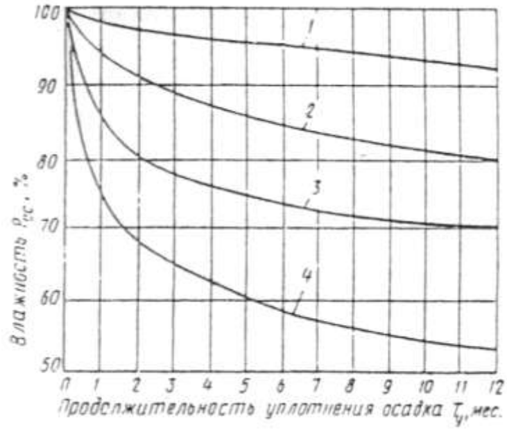
Рис. 4. Средние значения влажности осадка станции обезжелезивания и реагентного умягчения воды при уплотнении до одного года 1 - реагентное обезжелезивание; 2 - безреагентное обезжелезивание; 3 - реагентное умягчение при магниевой жесткости более 25%, 4 - реагентное умягчение при магниевой жесткости менее 25%
